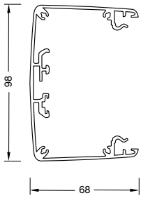
tehalit.DA 200 (1-fach)
