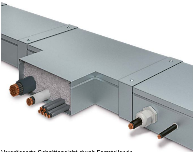
Vergrosserte Schnittansicht durch Formteile
