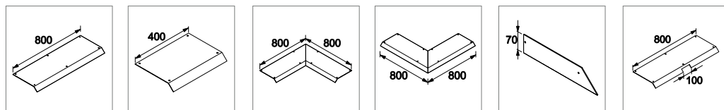
Blinddeckel Länge 800 mm Stahlblech
