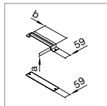
Kupplung Stahlblech
