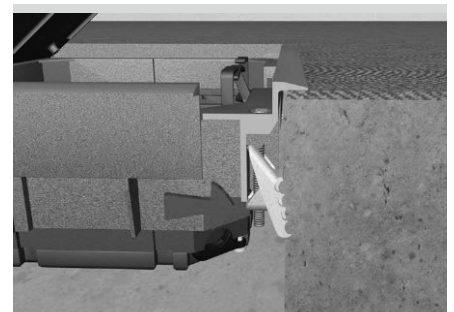
Einbau in Hohlböden
