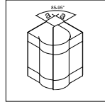
Ausseneck verstellbar ±5°
