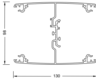
tehalit.DA 200 (2-fach)
