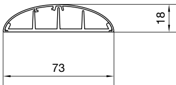
Aufbodenkanal SLA 18075 SL 18075
