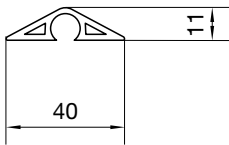
Aufbodenkanal SL 11040
